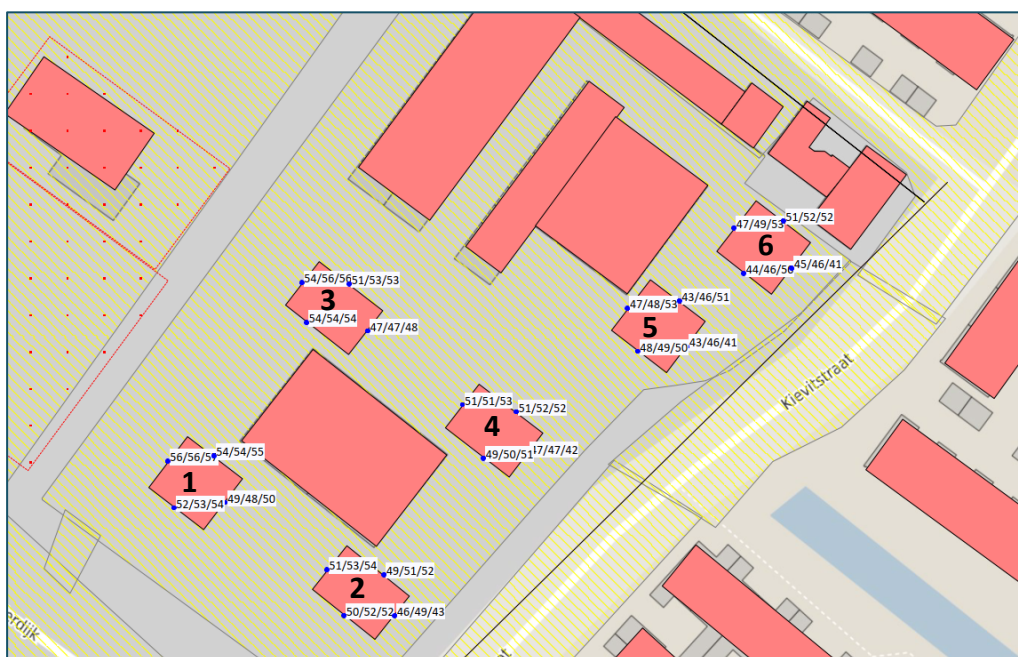
Figuur 8 Geluidsbelastingen volgens zonemodel met uitbreiding 'lege' kavels op basis van huidige milieucategorie
