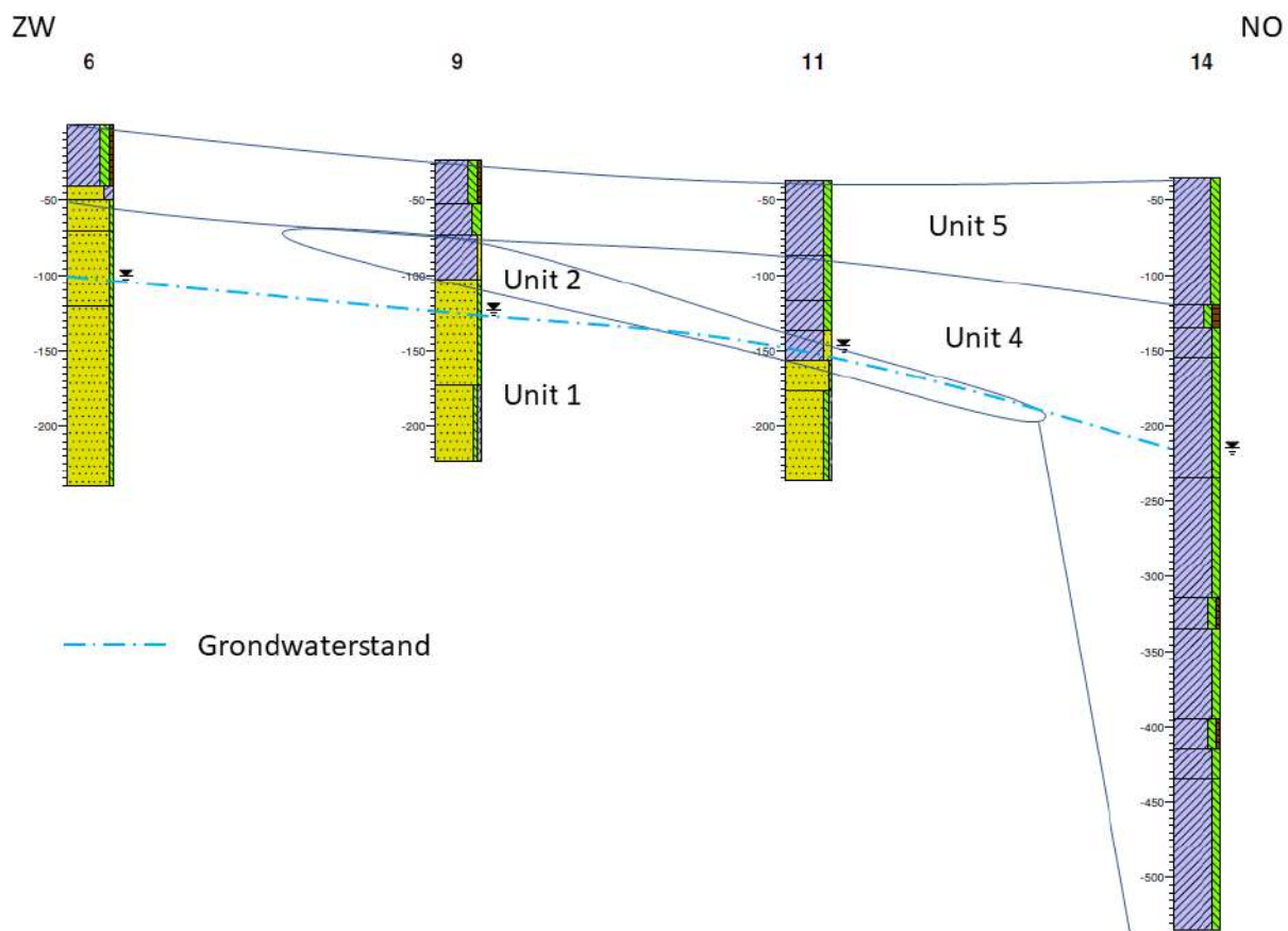
Figuur 11: ZW – NO profiel van het plangebied (profiel 1). Voor de locatie van profiel 1 binnen het plangebied zie Figuur 10. Voor de legenda zie Bijlage 4.
