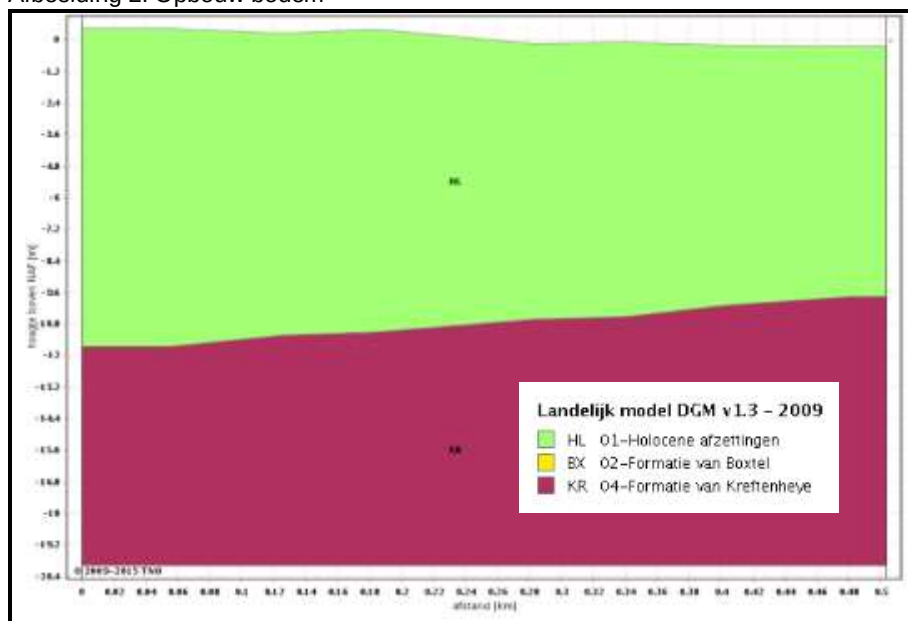
Afbeelding 2: Opbouw bodem
