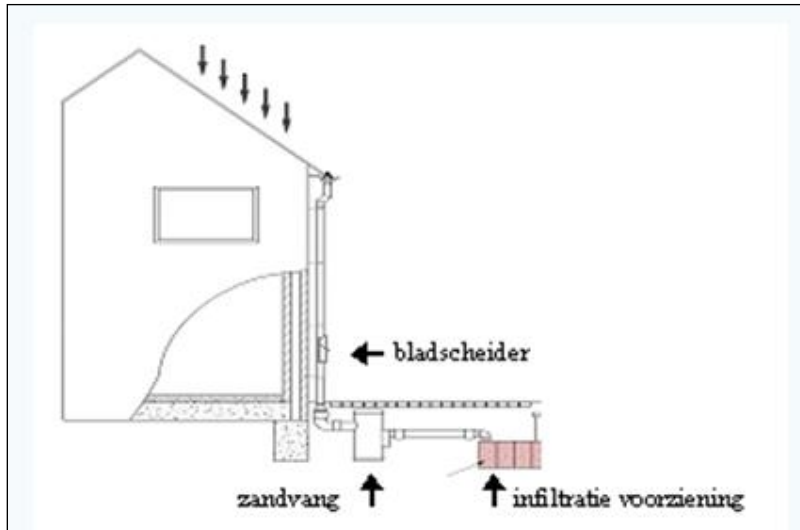
Afbeelding 4.2: Schematisch voorstelling infiltratievoorziening met elementen(infiltratiekragen).
