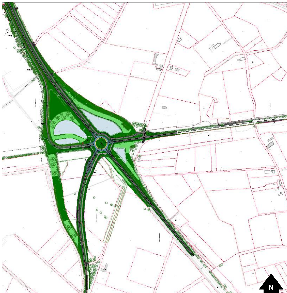
Figuur 4.1: reconstructieontwerp aansluiting N275-N277-N562
