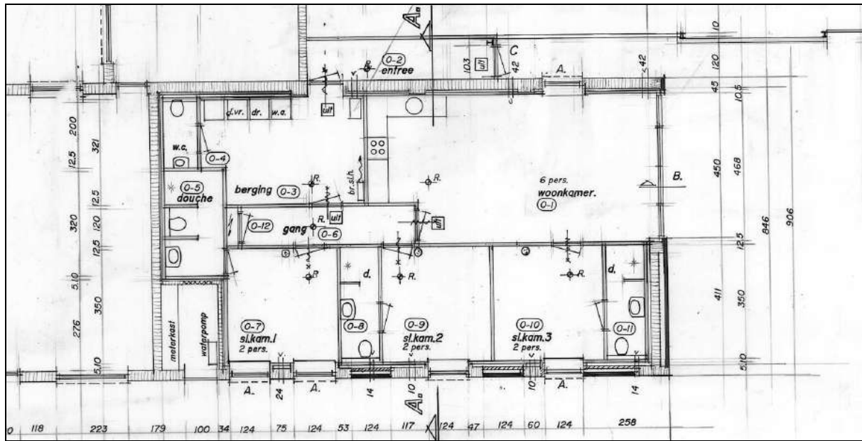
Figuur 6. Bouwtekening huisvesting 6 stagiaires
