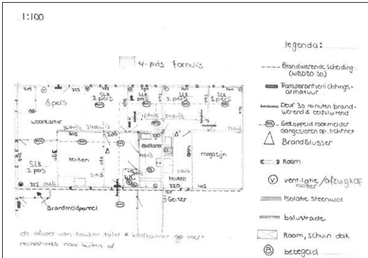
Figuur 6. Bouwtekening huisvesting 8 arbeidskrachten
