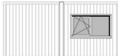
Zijaanzicht (schaal 1:100)
