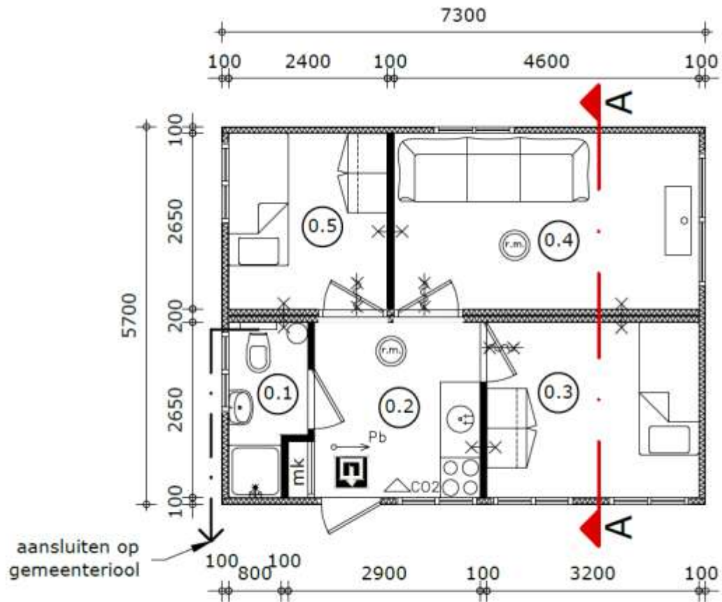
Plattegrond unit (schaal 1:100)
