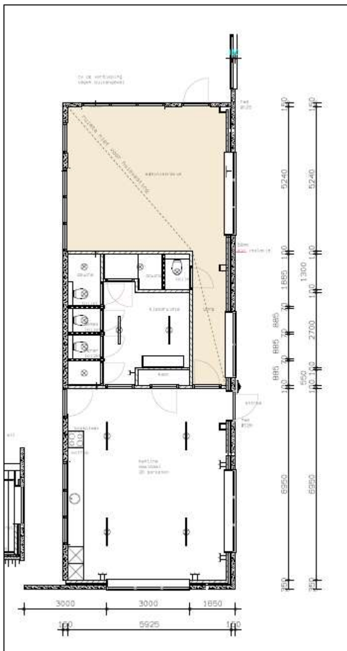
Figuur 7. Bouwtekening in pandige verbouwing bedrijfsloods
