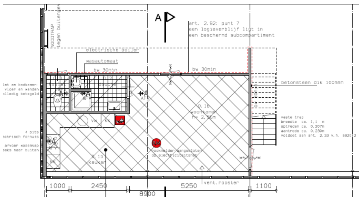
Figuur 6. Bouwtekening huisvesting 6 arbeidskrachten, begane grond
