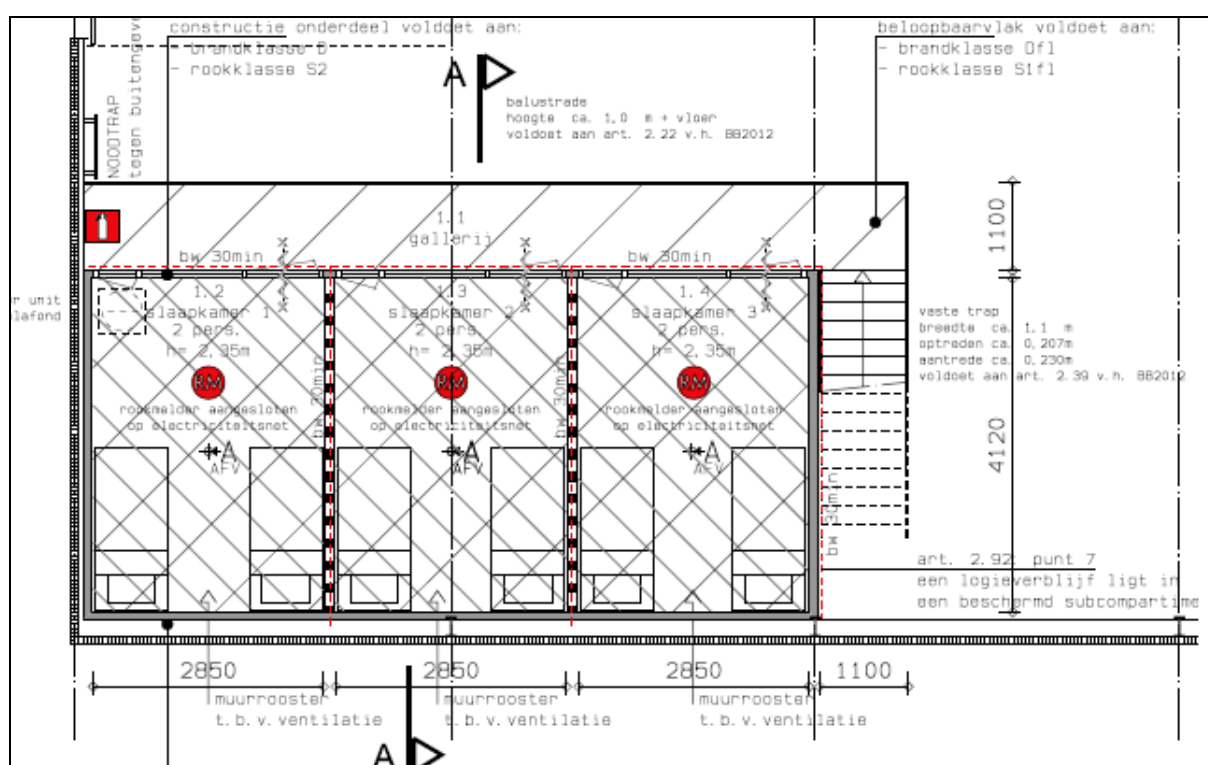
Figuur 7. Bouwtekening huisvesting 6 arbeidskrachten, verdieping
