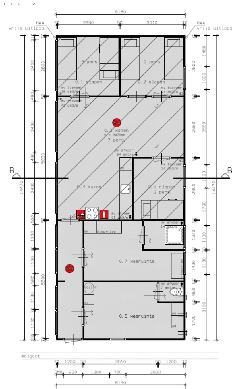
Figuur 6. Bouwtekening Huisvesting 17 tijdelijke arbeidskrachten in bedrijfsbebouwing
