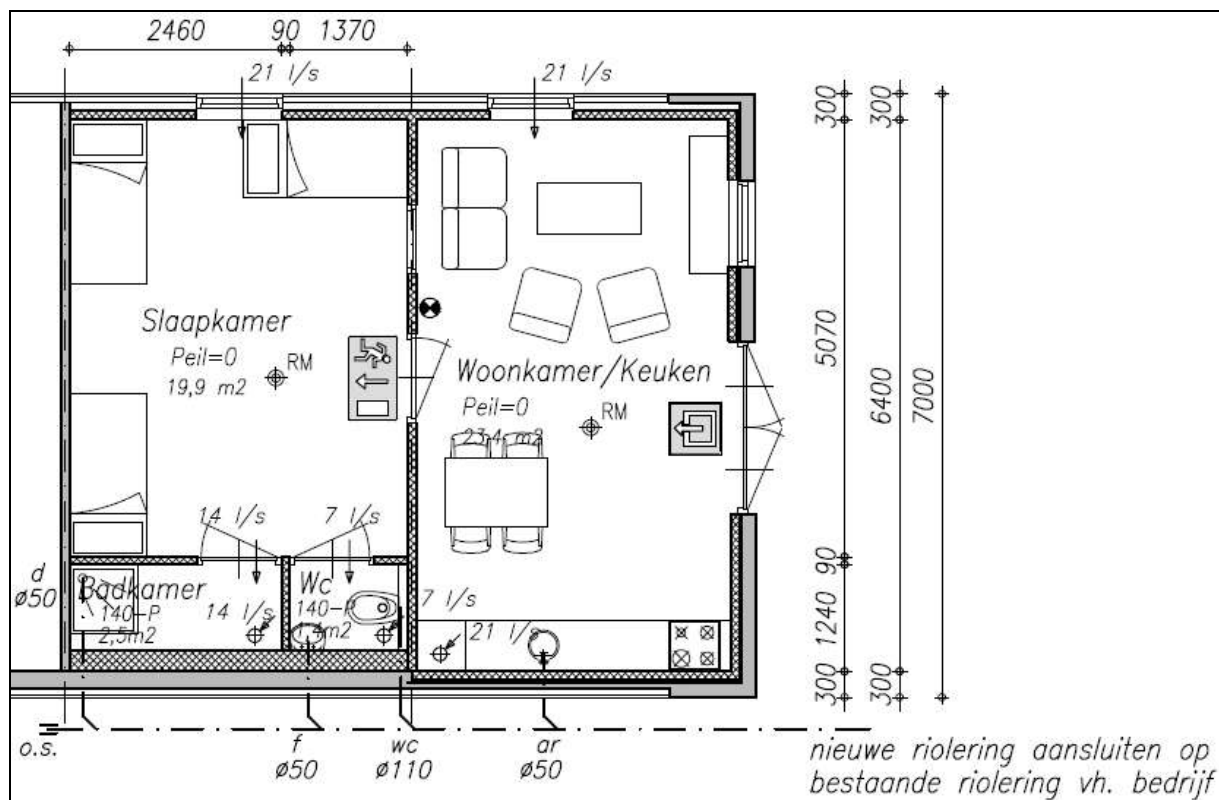
Figuur 6. Bouwtekening huisvesting
