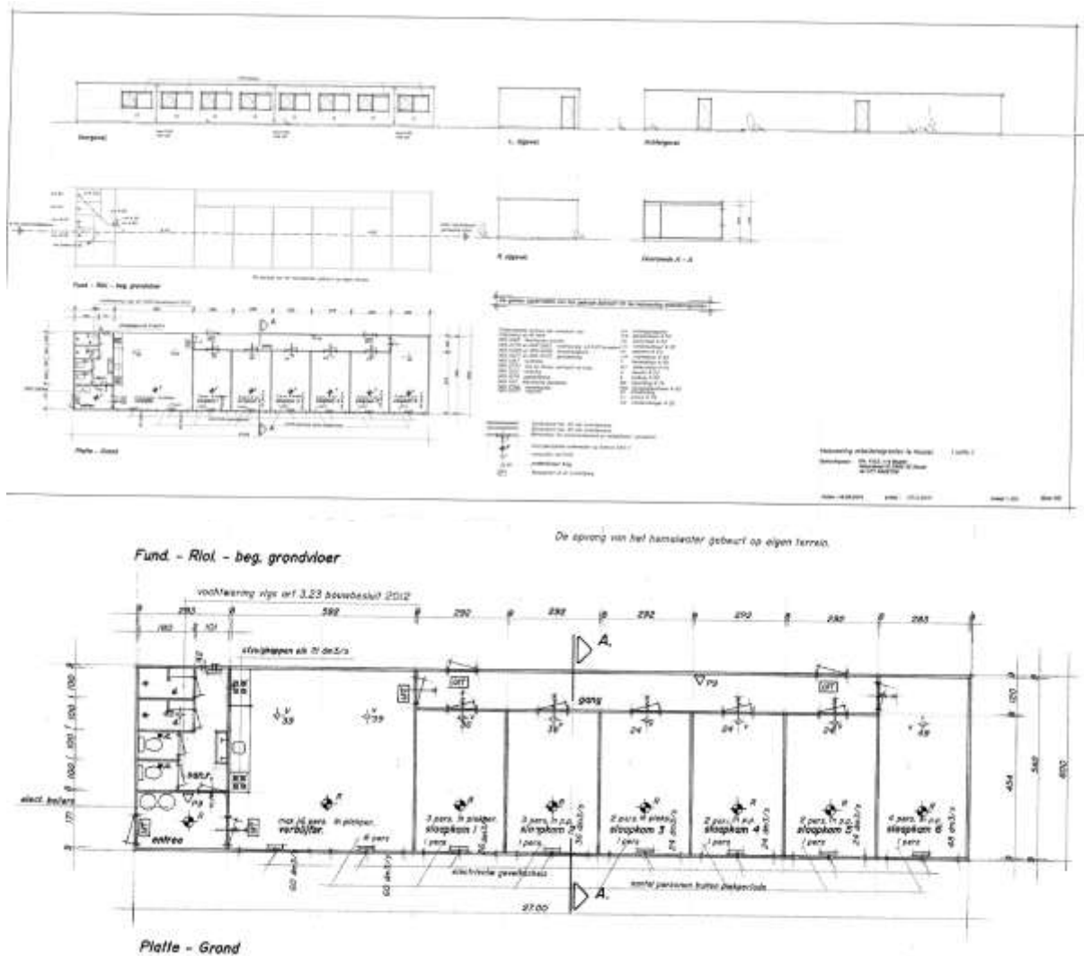
Figuur 6. Bouwtekening huisvesting
