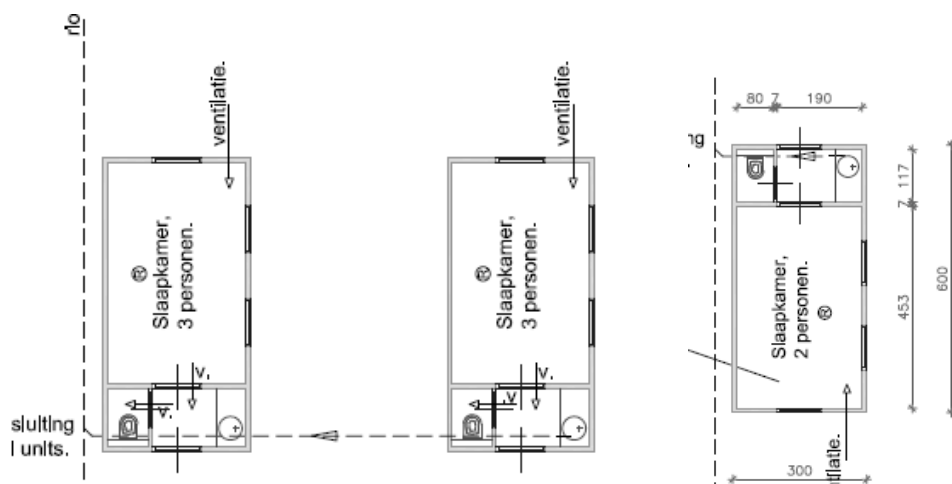
Figuur 6. Bouwtekening van de drie units waar de slaapkamers aanwezig zijn.
