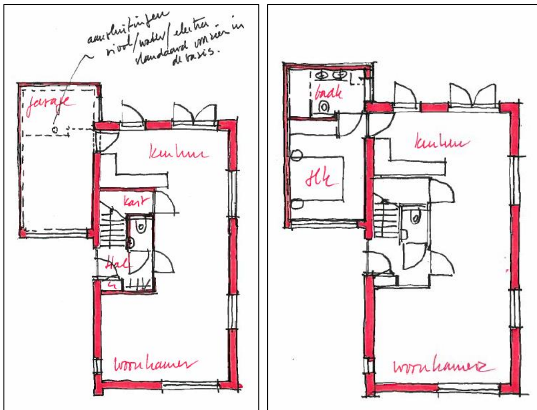
Schets basis type woning regulier (links) en levensloopbestendig (rechts)
