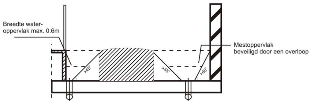
Doorsnede B-B
