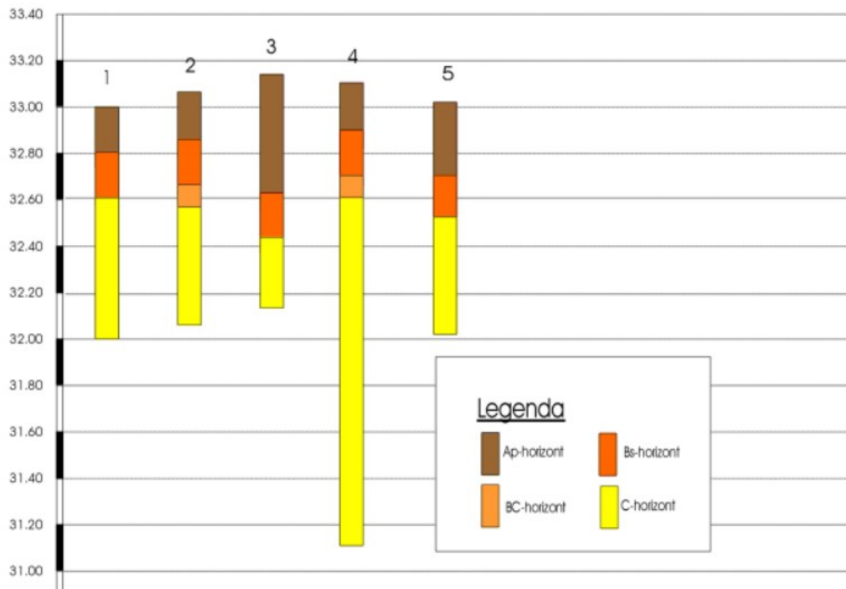
Figuur 18: Boorprofielen
