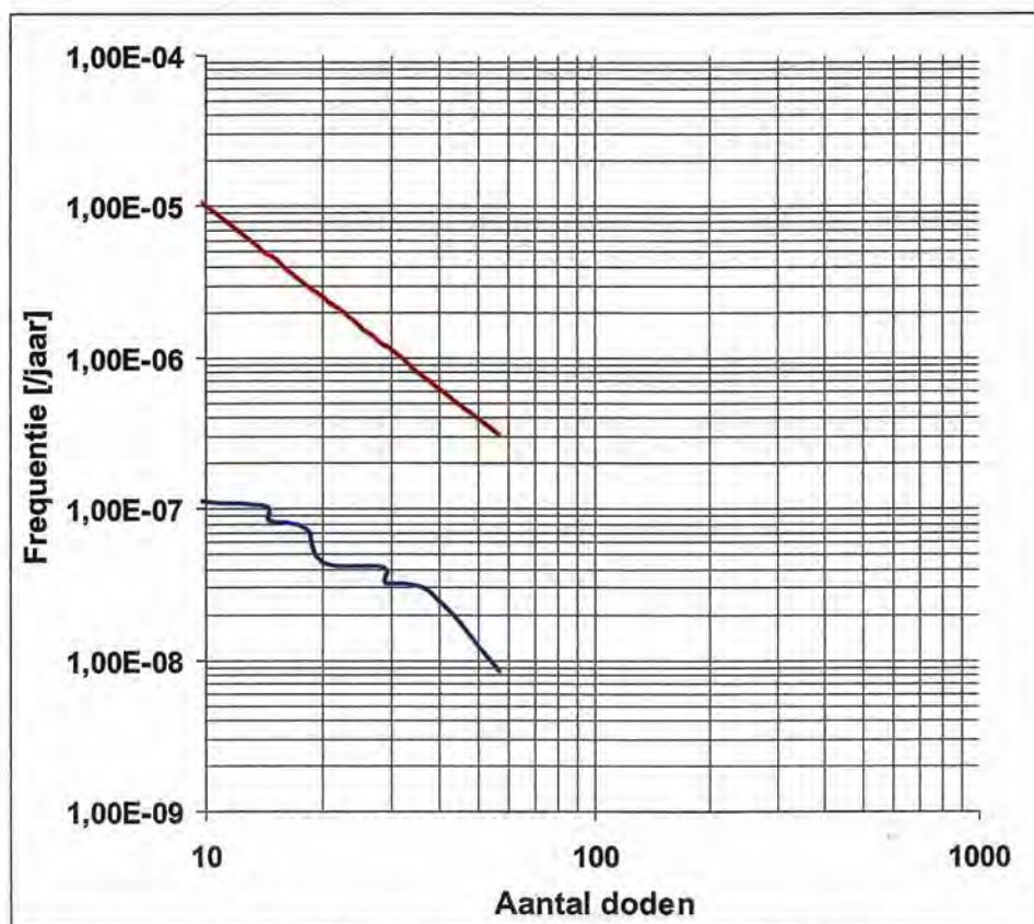
Figuur 1: fN-curve groepsrisico Van Hal met doorzet 500 m 3 /jaar
